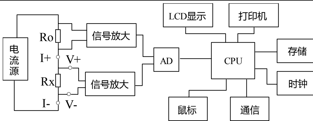
图 2 测试原理图
