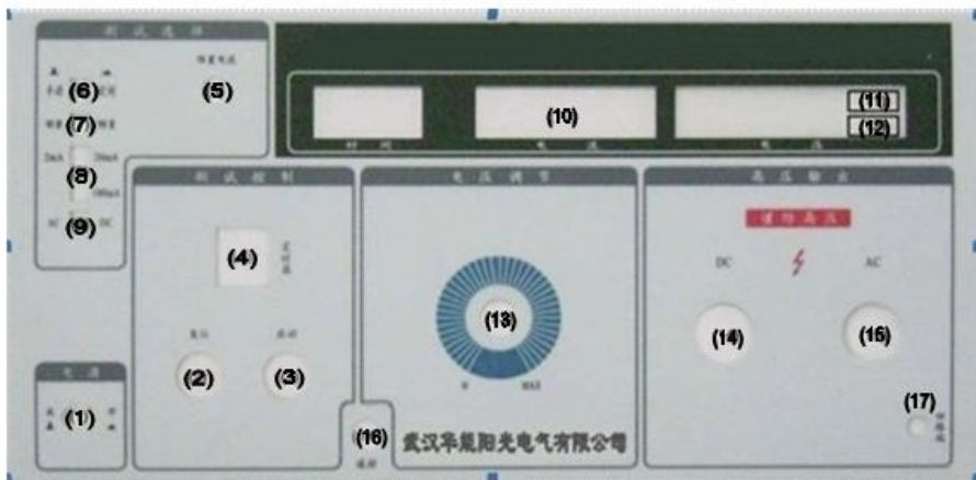
图 (2) HYG2670D 耐压测试仪前面板示意图
