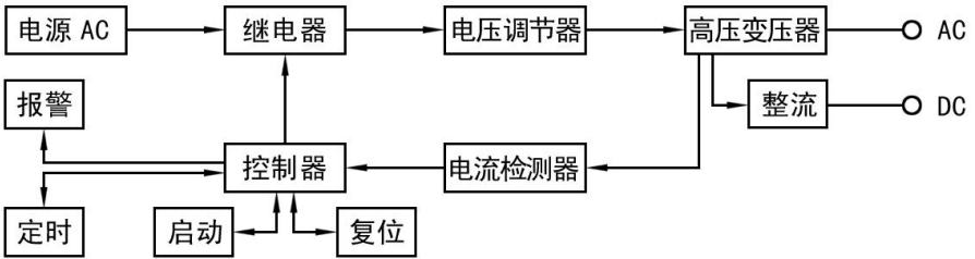
图(1):HYG2670E 耐压测试仪工作原理方框图
