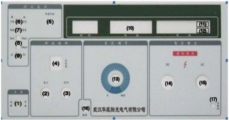
图（2）HYG2670E 耐压测试仪前面板示意图
