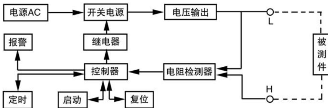
HYG2675D-II 绝缘电阻测试仪工作原理框图
