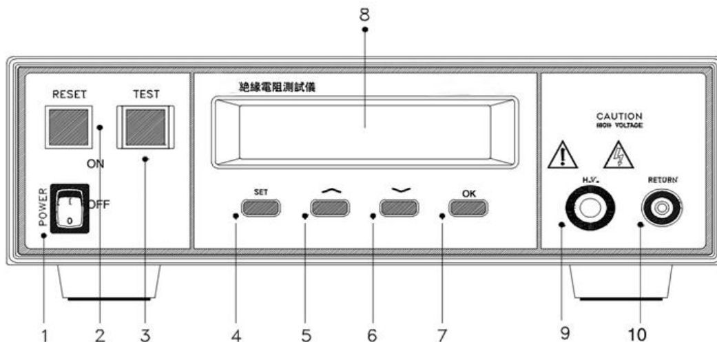
图（1）HYG2675D-II 程控绝缘电阻测试仪前面板示意图
