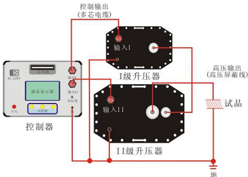
图 4 （连线图）
