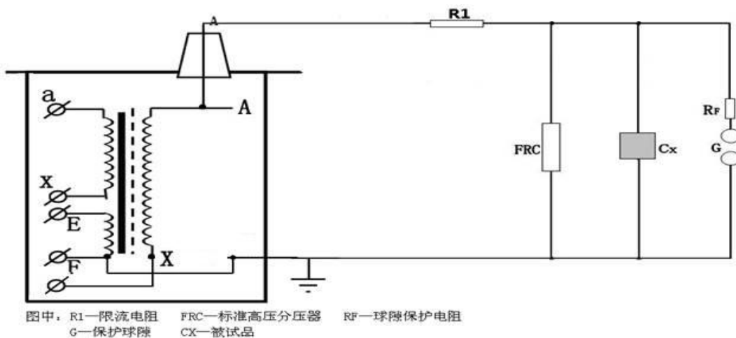
图3 工频耐压试验原理图
