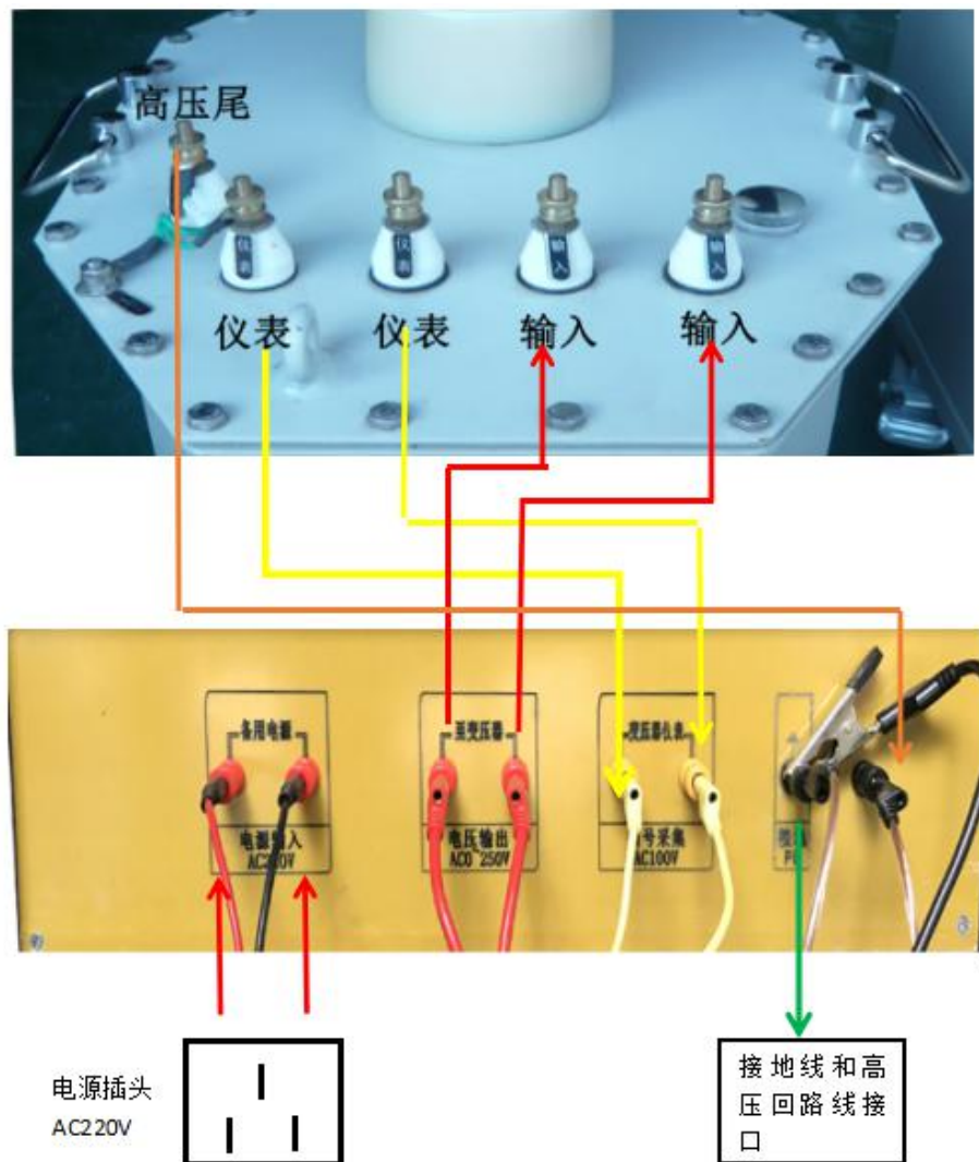
图 4 接线图
